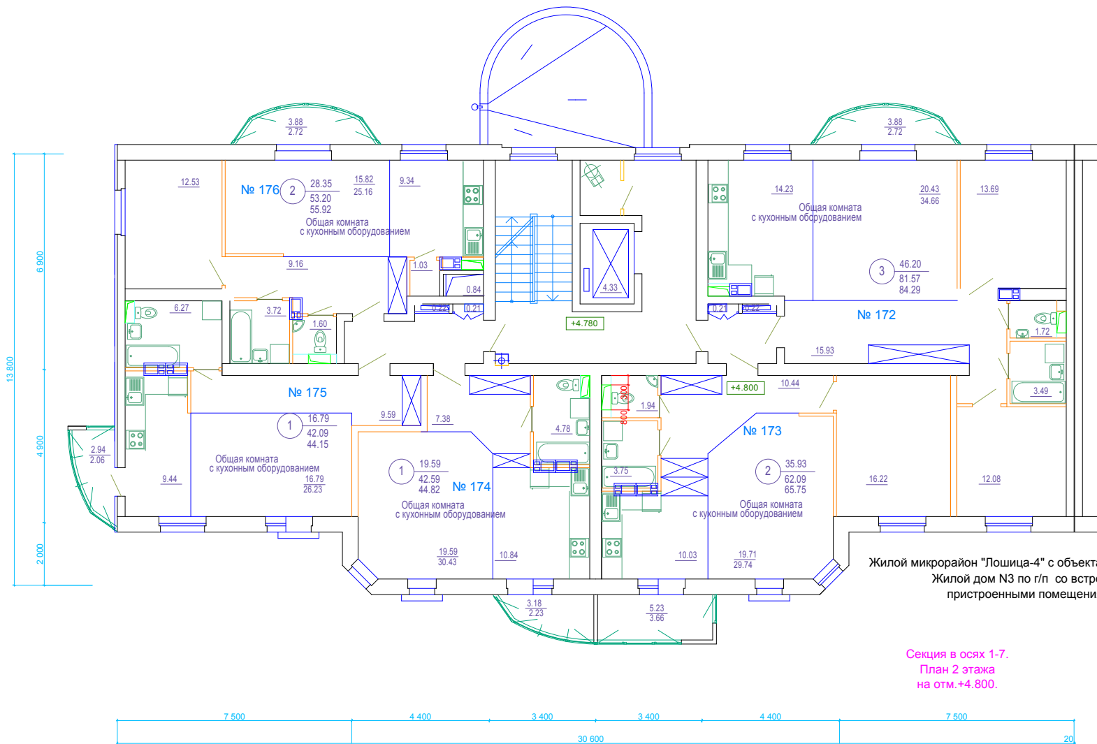
СХЕМА ПЛАНА
